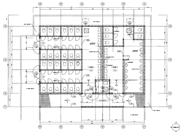
平面詳細図 1/50
