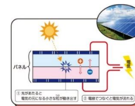
太陽電池の仕組み 出典:資源エネルギー庁WEBサイト
