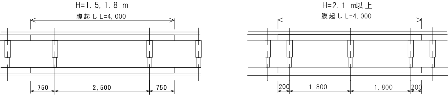
支保工平面図
