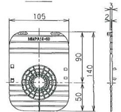
⑧ 土留板
