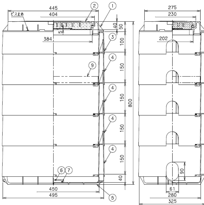
( 図 - 6 - 1 ) ヌ一タ一筐 ( \phi 13 \sim \phi 25 )
