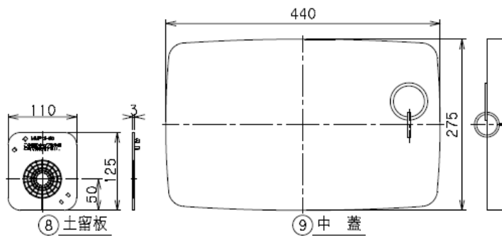
平面图
