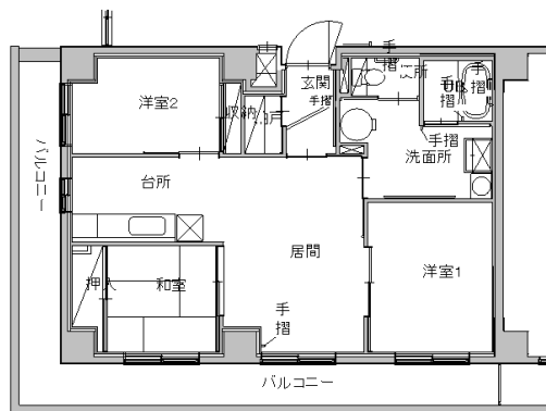
平面詳細図1 (3LDK-G1・G2)
