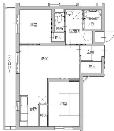
住戸平面図 2LDK-1C (1階)
