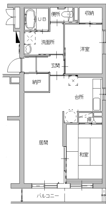
住戸平面図 2LDK-1A (2～5階)
