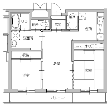
住戸平面図 2LDK-2B (2～5階)
