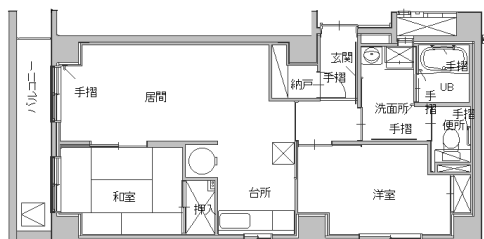
平面詳細図3(2LDK)
