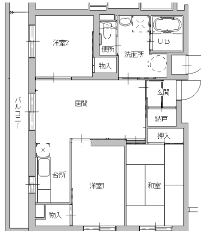
住戸平面図 3LDK (2～5階)
